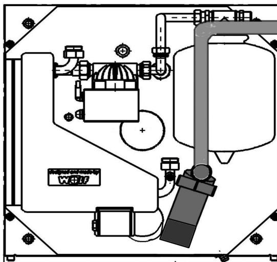
Draufsicht CS
