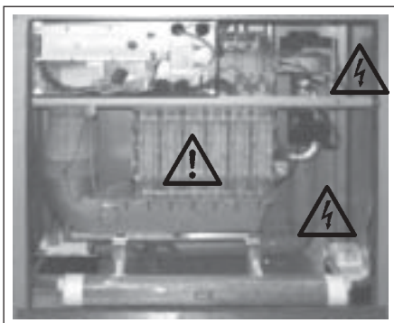
Bild: Zündtrafo, Hochspannungs- Zündelektrode, Ionisationselektrode, Wärmetauscher, Gefahr durch elektrische Spannung, Gefahr durch Verbrennung durch heiße Bauteile
