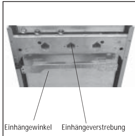
Bild: Gastherme in Einhängewinkel einhängen
