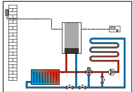
Bild: Fußbodenheizung
