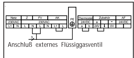
Bild: Anschluß externes Flüssiggasventil
