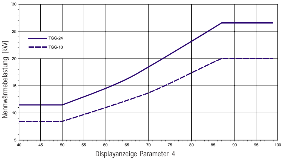
Diagramm: Nennwärmebelastung
