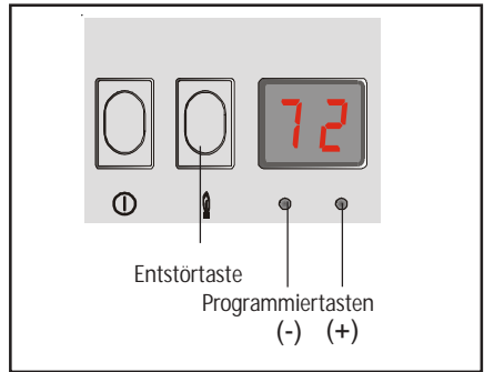
Bild: Programmier Tasten
