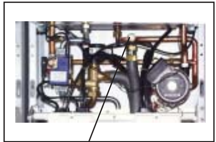
Bild: Entlüfterschraube Heizkreis
