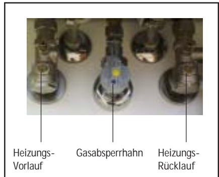
Bild: Absperrarmaturen
