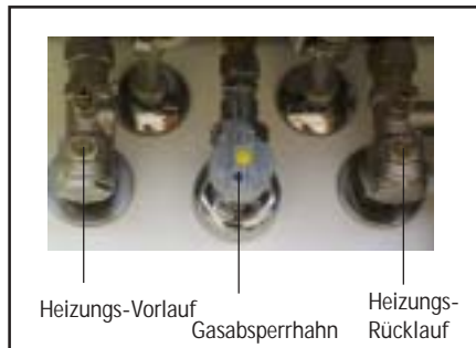
Bild: Absperrarmaturen
