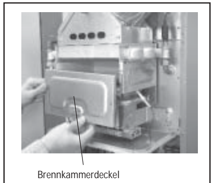
Bild: Brennkammerdeckel
