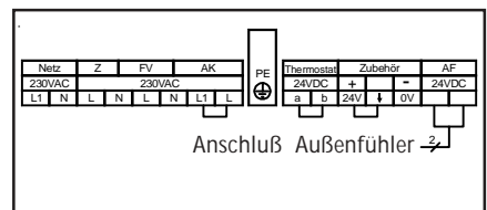
Bild: Anschluß Außenfühler
