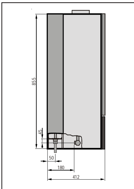
Bild: Abmessungen
