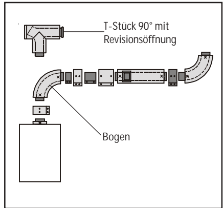
Bild: Rohrlängenberechnung
