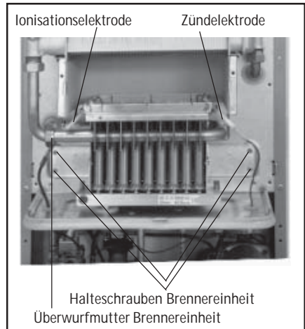
Bild: Brenneinheit ausbauen
