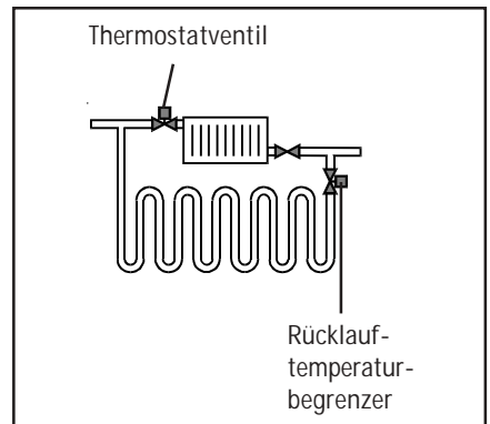
Bild: Fußbodenheizung
