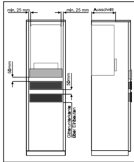
Bild: Schrankeinbau
