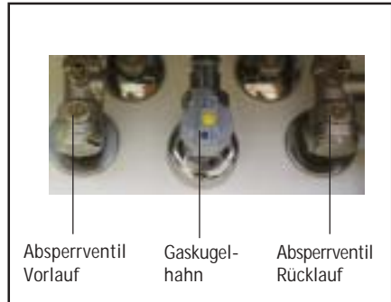
Bild: Absperrreinrichtungen
