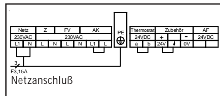
Bild: Netzanschluß
