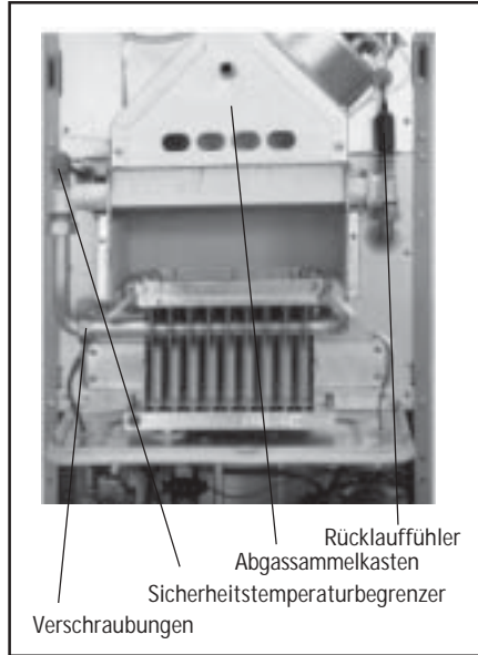
Bild: Demontage Heizwasserwärmetauscher
