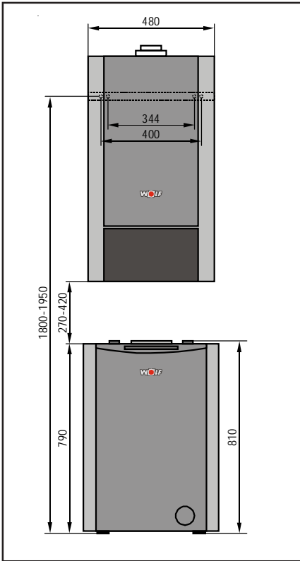
Bild: TGG mit TSW-120 ohne Blende für Verrohrung
